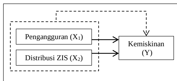
Gambar 3. Kerangka Konseptual
